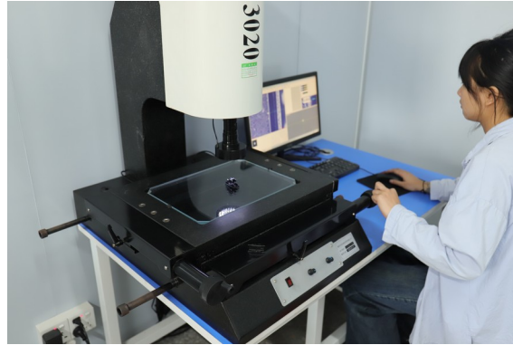
2 차원 측정기
