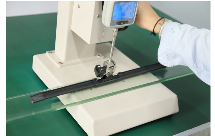
압력 시험기
